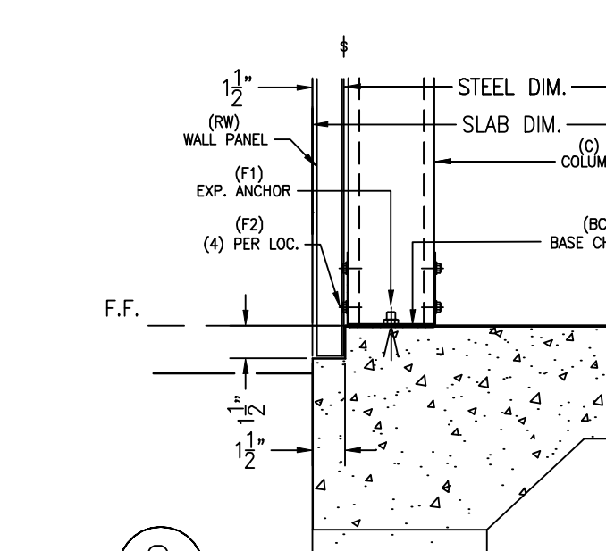
2 WALL EDGE BASE
