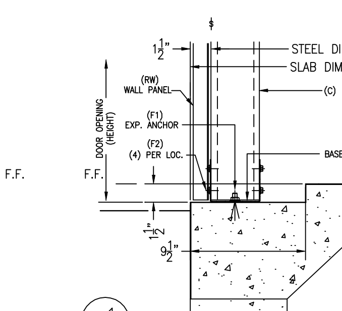
1 DOOR EDGE BASE
